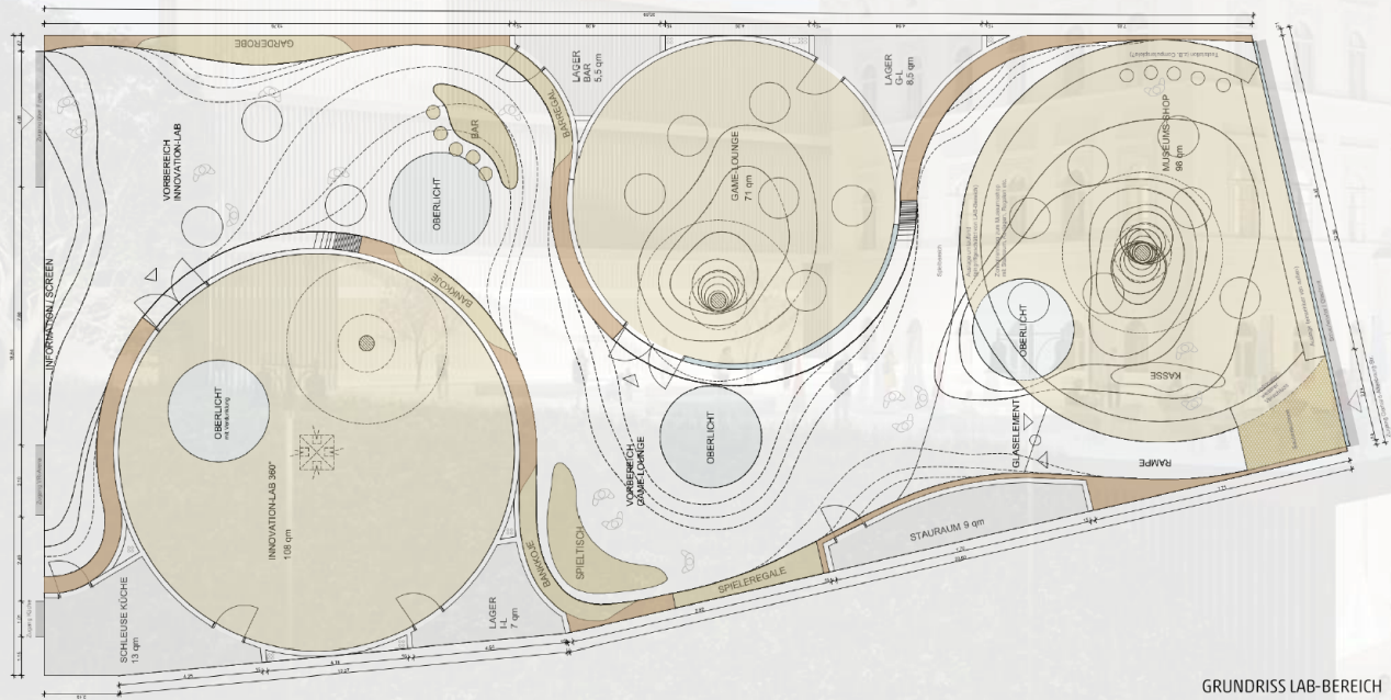
GRUNDRISS LAB-BEREICH
